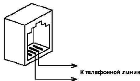
Рис. 2.2. Подключение телефонной линии
