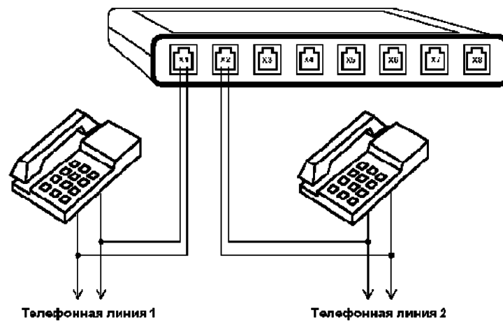
Рис. 2.1. Подключение адаптера к телефонной линии
