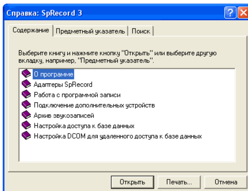
Рис. 2.10. Содержание справки
